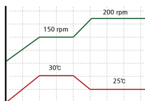
◀12 Program 온도, 속도 설정 가능 Fix / Program mode 운전 가능
